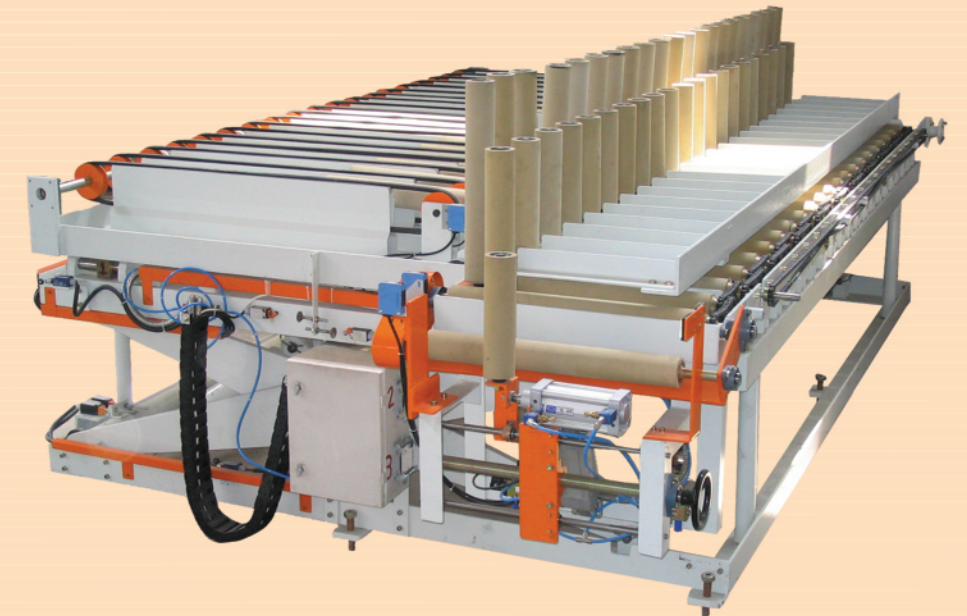
PANEL BOŞALTMA ve YATIRMA KONVEYÖRÜ Panel Unhooking and Driving Conveyor
